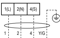
Наружные блоки
